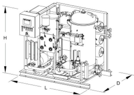
ULTRA-SEP 7500 & 10000
