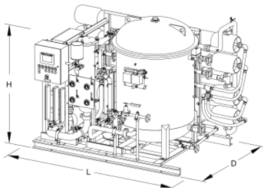
ULTRA-SEP 7500 & 10000
