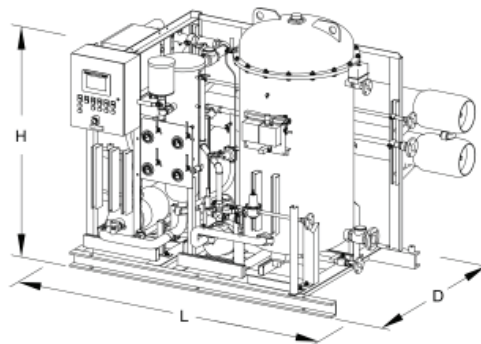
ULTRA-SEP 5000
